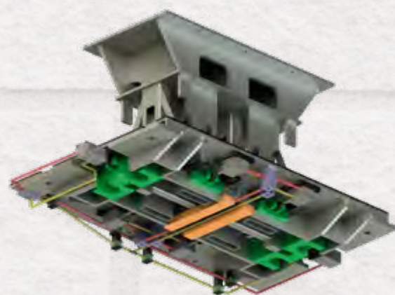
MOLDE HIDRAULICO
